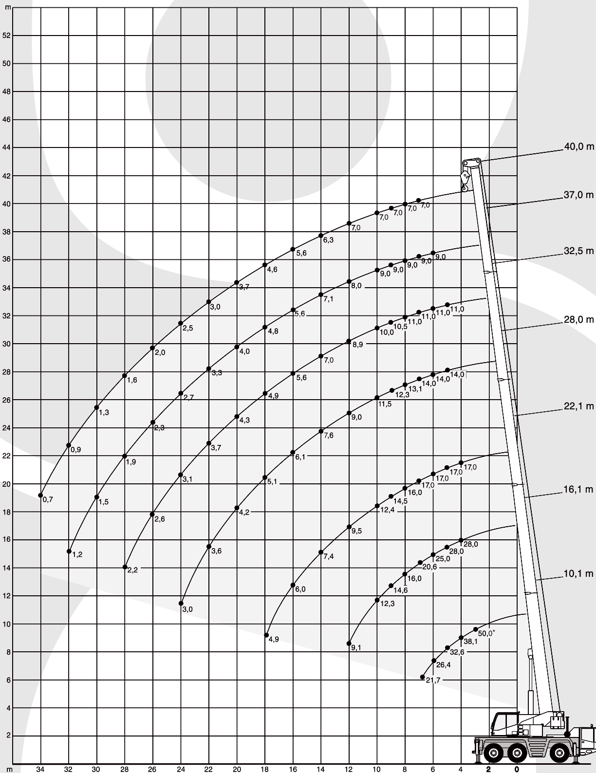
Zasięg pracy: wysięgnik podstawowy
